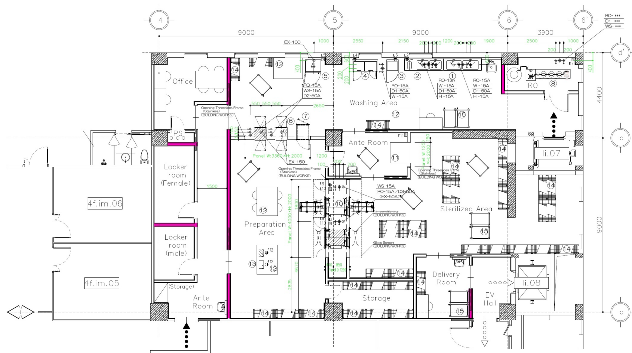
Một mặt bằng phân khu đơn vị tiết khuẩn trung tâm mà JVC và Sakura Seiki đã thiết kế cho khách hàng
